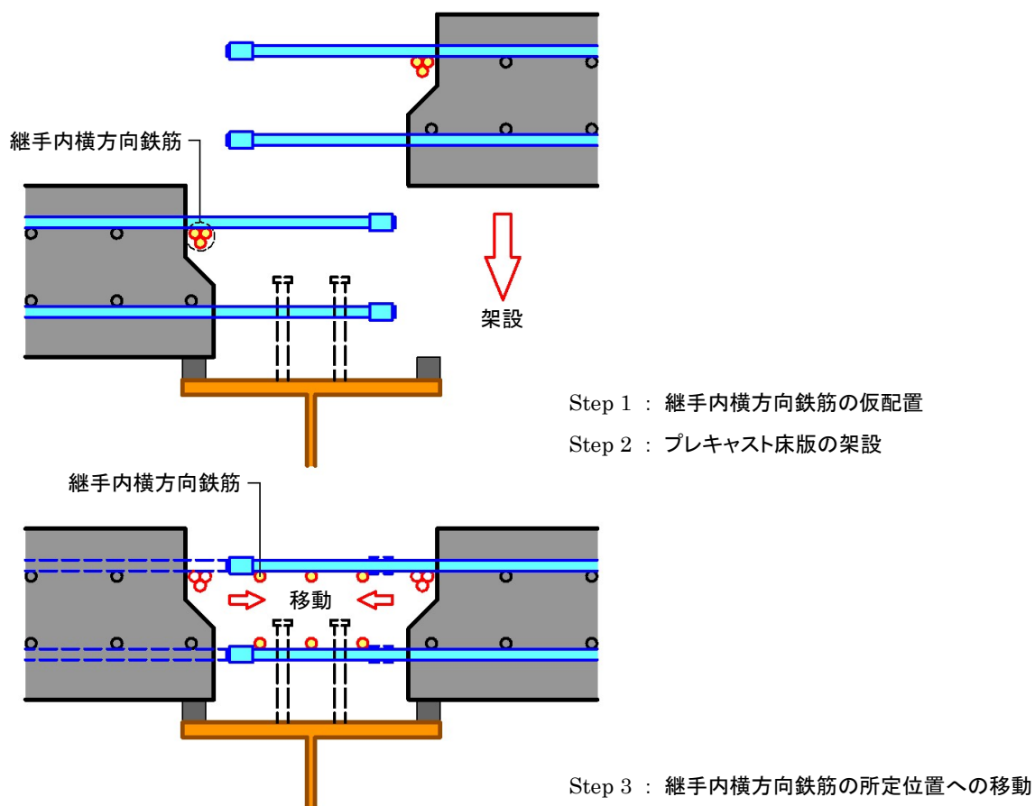
【SLJスラブの架設手順】
