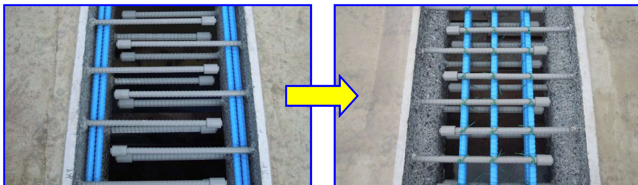
【継手内横方向鉄筋の配置手順 Step 3】
